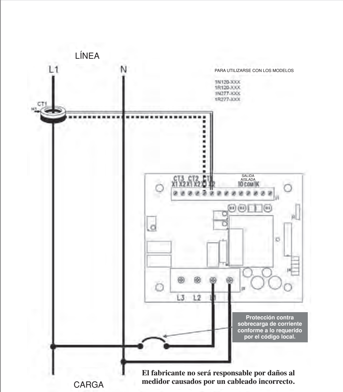
Figura 7: Diagrama del Sistema de Conexión de 1 Fase, 2 Cables
