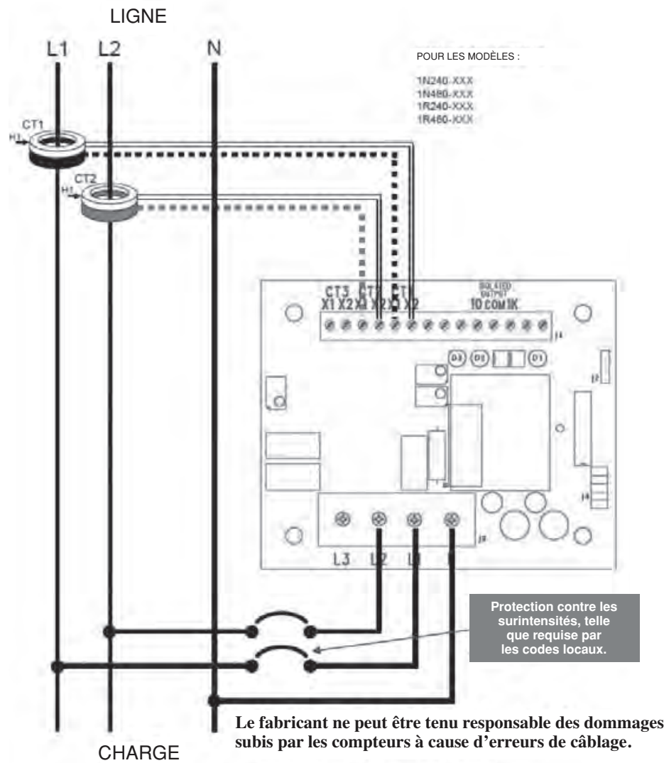
Figure 8 : Installations monophasées ou biphasées trifilaires
