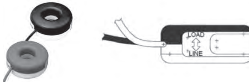
Figura 5: TC de Núcleo Sólido de Leviton
