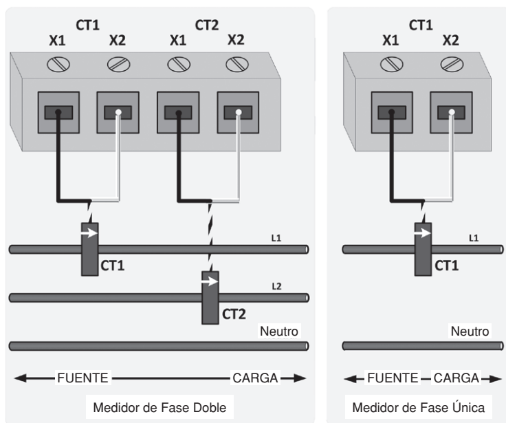
Figura 6 – Diagrama de Cableado del TC
