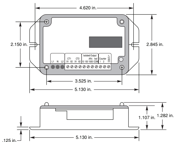
Figure 1 - Single Mini Meter Case Dimensions
